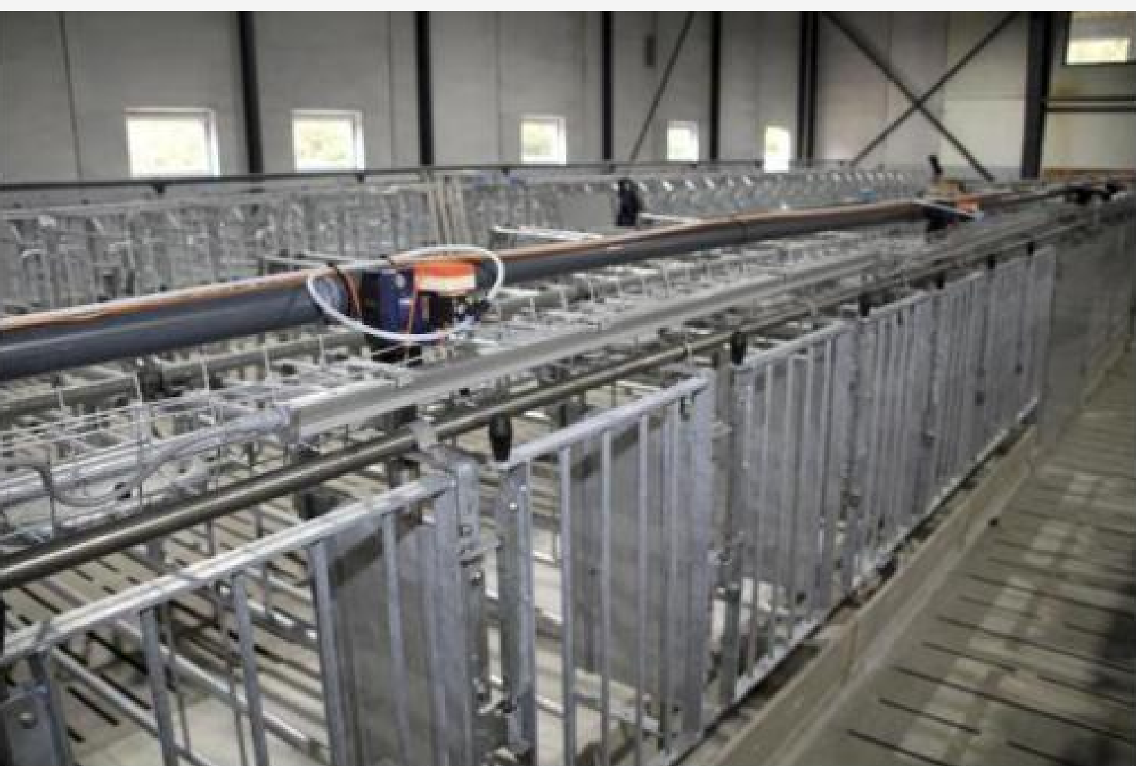
Hier ein weiterer Einblick, wie das LED-Licht parallel zur Zuleitung verläuft, die einspeisen kann einzeln bis auf drei oder vier Seen. Zu diesem Zweck werden Teile des Futterstrangs unterhalb des Bodenniveaus verlegt gute Sicht auf die Scheune.
